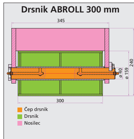
Tip: 8756-C Čep drsnik 31,93 € Tip: 8756-R Drsnik 43,26 € Tip: 8756-D Nosilec 26,78 €
