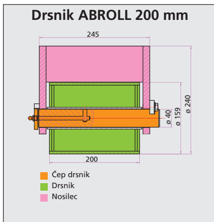
Tip: 8709-C Čep drsnik 26,78 € Tip: 8709-R Drsnik 35,02 € Tip: 8709-D Nosilec 25,75 €
