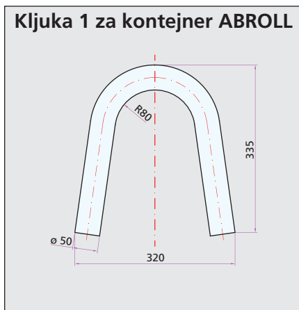
Tip: 8753-1 Kljuka 1 za kontejner ABROLL 53,56 €
