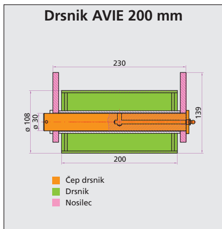
Tip: 8788-C Čep drsnik 18,54 € Tip: 8788-R Drsnik 26,78 € Tip: 8788-D Nosilec 25,75 €
