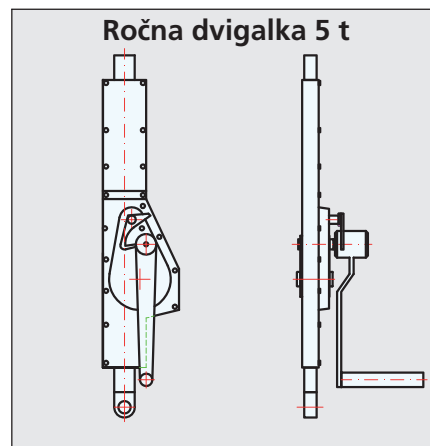
Tip: 8841 Ročna dvigalka 5 t 473,80 €
