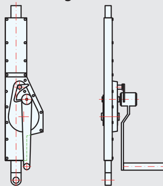
Ročna dvigalka 2,5 t
