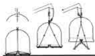
Sistem praznjenja A – Primeren za zbiranje steklene in plastične embalaže.
