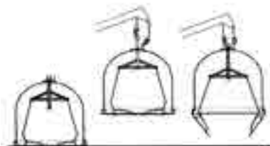
Sistem praznjenja B – Primeren za zbiranje papirja, stekla in plastične embalaže.
