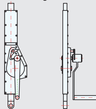
Ročna dvigalka 5 t
