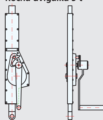
Ročna dvigalka 5 t
