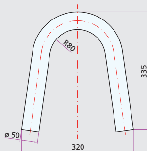
Kljuka 1 za kontejner ABROLL
