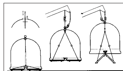
Sistem praznjenja A – Primeren za zbiranje steklene in plastične embalaže.
