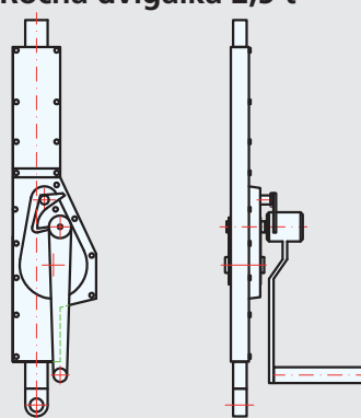
Ročna dvigalka 2,5 t
